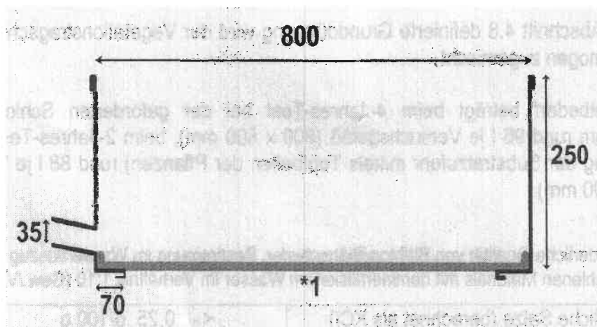
Abb. 5: Aufbau der Versuchsgefäße (Mindestmaße, Angaben in mm, *1 = transparenter Boden mit Aufkantung)
