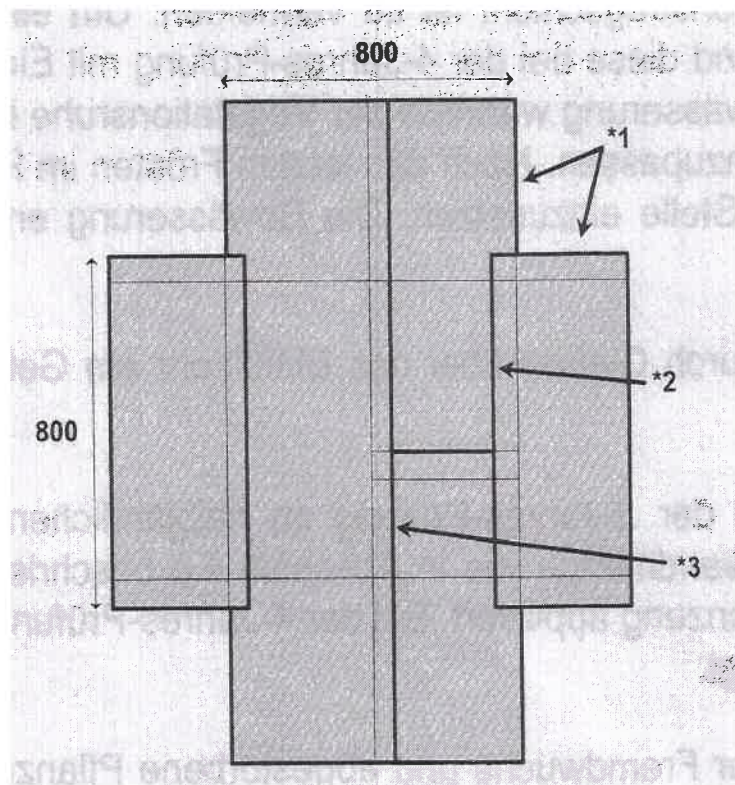
Abb. 7: Anordnung der Nähte (*1 = Wand-Ecknaht, *2 = Boden-Ecknaht, *3 = T-Naht) in der zu untersuchenden Bahn (Maße in mm).
