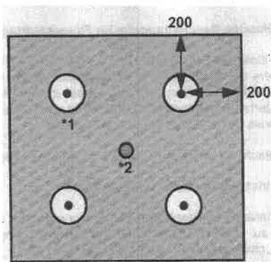
Abb. 6: Anordnung der Gehölze (*1) und des Tensiometers (*2) in der Vegetationstragschicht bei einem Gefäß von 800 x 800 mm (Maße in mm)
