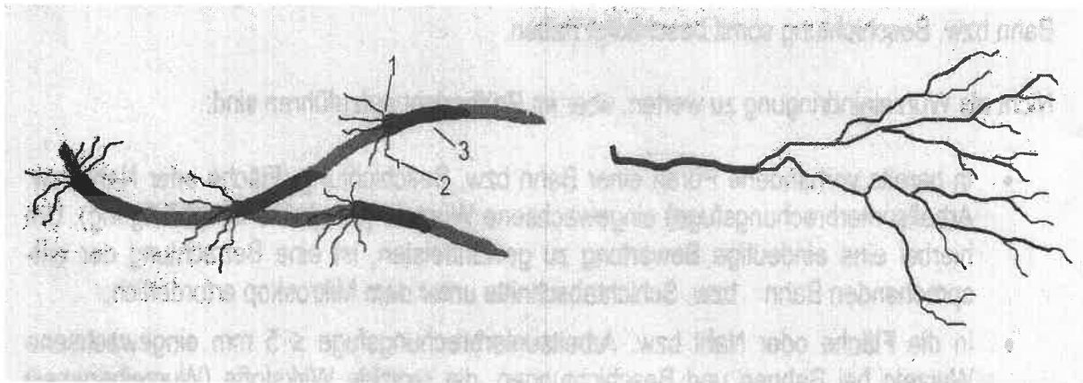
Abb. 4: Schematische Darstellung eines Quecken-Rhizoms (links) mit Knoten (1), Wurzeln (2) und Blättern (3) im Vergleich zu einer Feuersporn-Wurzel (rechts)
